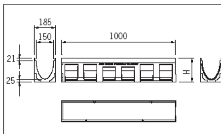
Desenho cotado do canal V 150, 1 m
