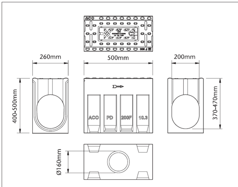
Canal de inspeção ACO Drain RoadDrain® 200, 0,5 m
